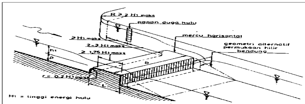
Gambar 3 Bangunan ambang lebar
