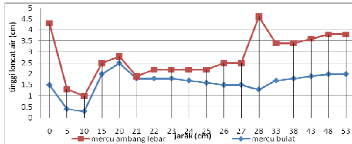
Gambar 9 Grafik Hasil Gabungan Perhitungan Tinggi Loncat Air Kolam Olak Pada Mercu Ambang Lebar Dan Mercu Bulat Q = 0,00027 \text{ m}^3/\text{dtk} So = 0
