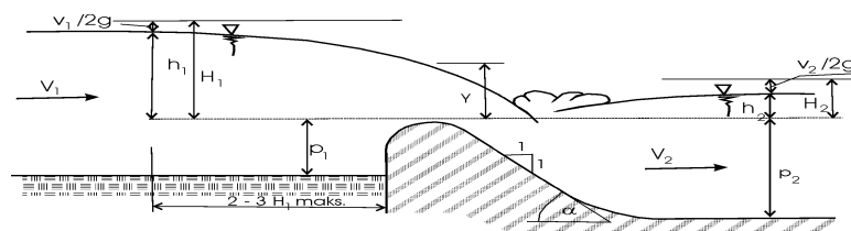
Gambar 2 Aliran melalui mercu bulat
