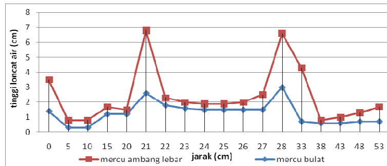
Gambar 8 Grafik Hasil Gabungan Perhitungan Tinggi Loncat Air Kolam Olak Pada Mercu Ambang Lebar Dan Mercu Bulat Q = 0,00027 \text{ m}^3/\text{dtk} S_0 = 2
