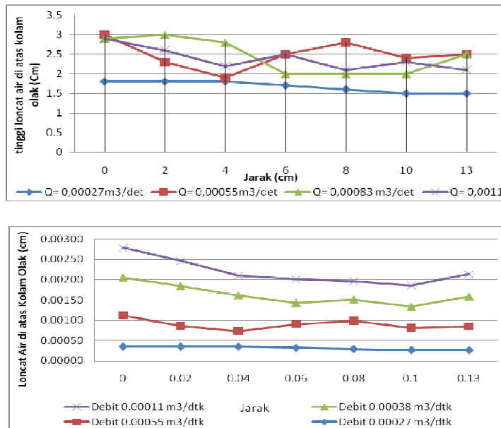
Gambar 6 Grafik simulasi laboratorium tinggi Loncat Air di atas Kolam Olak Pada Mercu Bulat, S_0 = 0
