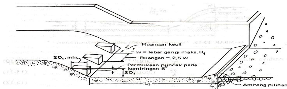
Gambar 4 Pembagian Kolam Olakan USBR IV.
