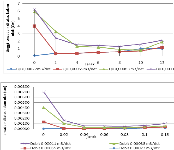
Gambar 7 Grafik Hasil Laboratorium Tinggi Loncat Air di atas Kolam Olak Pada Mercu Ambang Lebar, S_0=0
