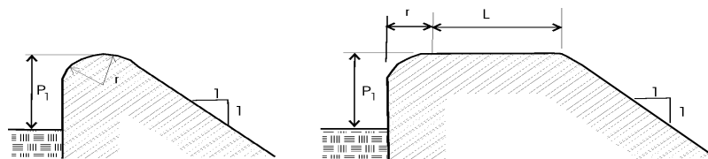
Gambar 1 Bentuk Mercu Bendung Tipe Bulat
