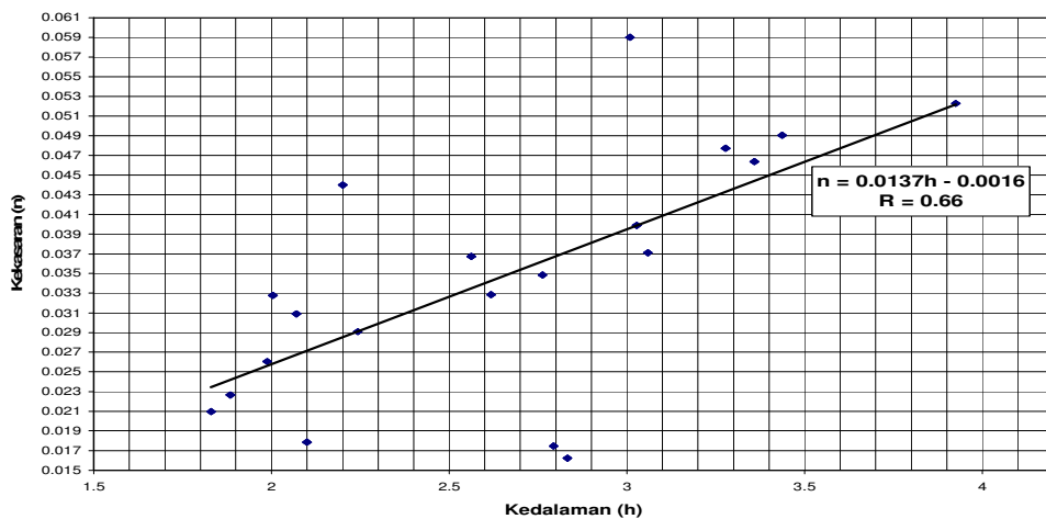
Gambar 1 Grafik hubungan kedalaman (h) terhadap kekasaran Manning (n)
